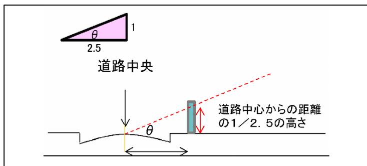
図 3-4 耐震診断義務付け対象の避難路沿道の組積造の塀
